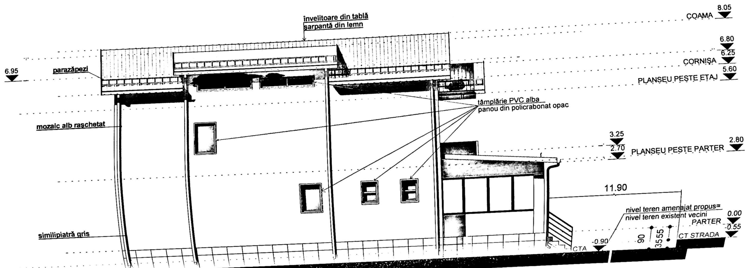
FAȚADA NORD-EST SC:1:100
